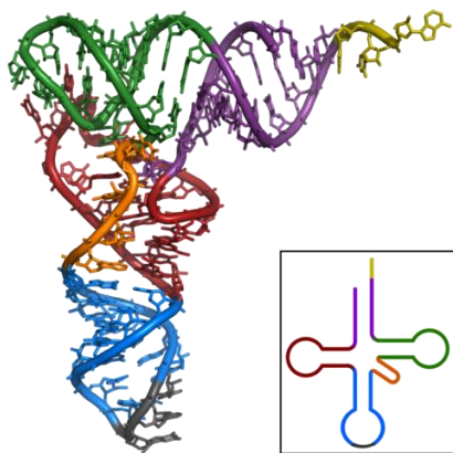
tRNA(Phe)
